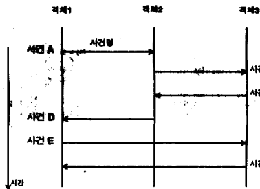
(그림 1) 사건 추적도 (Fig. 1) Event Trace Diagram
