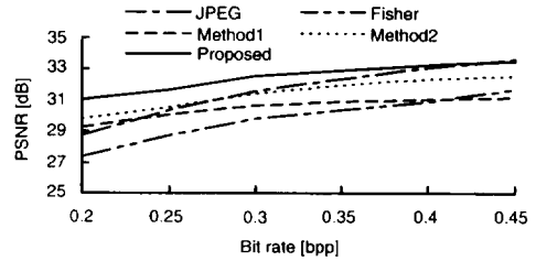
(그림 3) 영상의 비트율 대 PSNR (a) LENA (b) PEPPER (Fig. 3) PSNR versus bit rate for images (a) LENA (b) PEPPER
