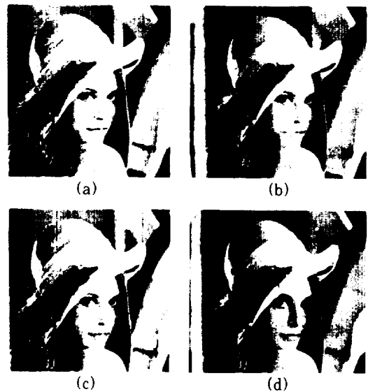
(그림 4) 0.30 [bpp]에서 LENA 영상에 대한 복원 영상 (a) JPEG 방법에 의한 복원 영상 (32.00 [dB]) (b) Fisher의 방법에 의한 복원 영상 (29.20 [dB]) (c) Krupnik의 방법에 의한 복원 영상 (31.04 [dB]) (d) 제안한 방법에 의한 복원 영상 (33.01 [dB])
