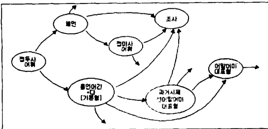
(그림 4-1) 한국어 형태소 해석결과에 의한 자연수화 형태소 생성규칙
