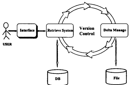
(그림 5) 시스템 모델의 구성 (Fig. 5) Structure of system model
