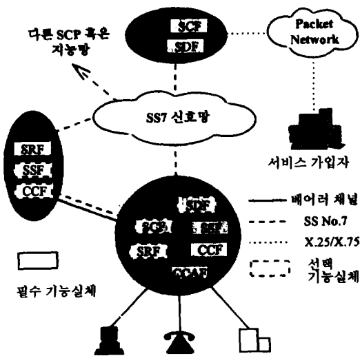
(그림 1) VOT 서비스를 위한 지능망 기능 구조 (Fig. 1) IN Functional architecture for televoicing service
