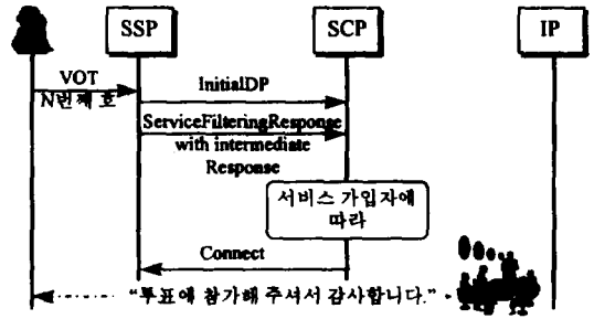
(c) 필터링 활성화 이후 N 번째 도착호의 경우 (c) When N-th call arrives in active filtering state
