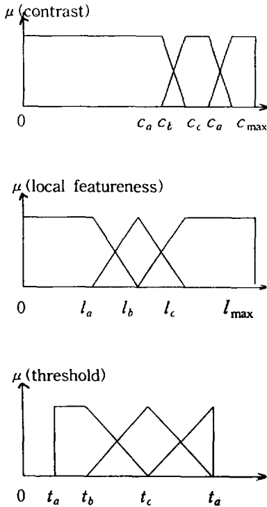
(그림 3) 입력 퍼지 소속함수
