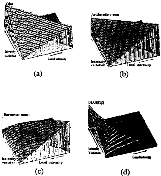
(그림 2) (a) 영상에서 나타날 수 있는 가능한 모든 현상 ; 및 (b) 산술평균의 출력 ; (c) 조화평균의 출력 ; (d) DBAH 연산자의 출력 특성
