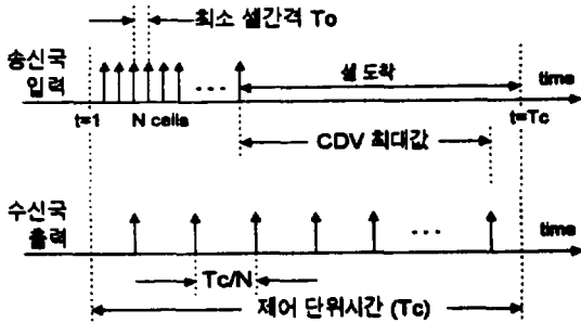
(그림 2) CDV를 최대로 하는 입력 패턴 (Fig. 2) Input pattern of CDVmax
