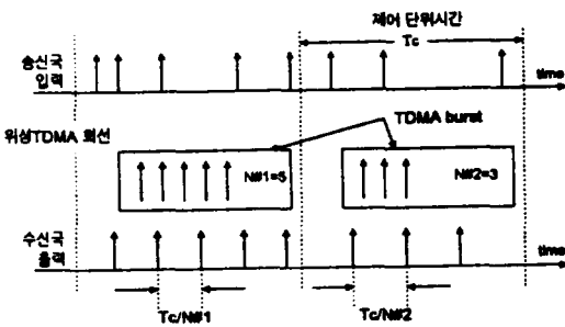
(그림 1) 셀 계수 방식의 개념도 (Fig. 1) Conceptual diagram of cell numbering method
