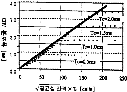
(그림 4) 포아송 분포의 CDV 분포폭
