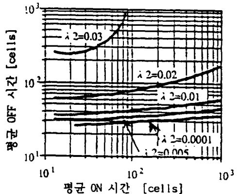
(그림 6) 최악 입력 패턴 발생 확률( 10^{-9} )의 영역 (Fig. 6) Region of worst case probability( 10^{-9} ) in input pattern
