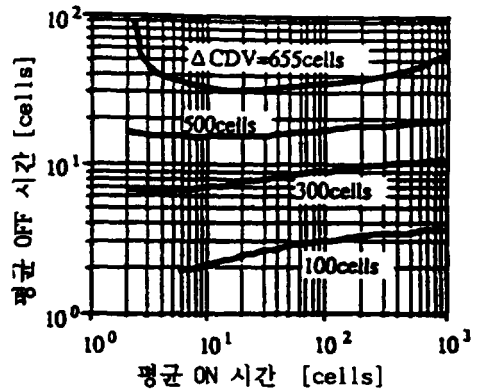
(그림 5) CDV 분포폭( 10^{-9} 값)의 분포(MMPP) (Fig. 5) Distribution of CDV distribution width( 10^{-9} )
