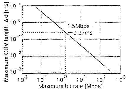
(그림 4) CDV 분포폭과 최대 전송속도의 관계 (Fig. 4) Maximum bit rate vs. maximum CDV length
