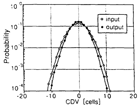
(그림 6) 제안 방식에서의 클러핑 보상 특성 (Fig. 6) Clumping compensation characteristic for proposed algorithm
