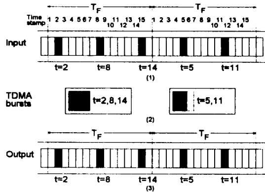
(그림 3) TDMA 링크에서의 타임 스탬프 방법 (Fig. 3) Time stamp method in satellite TDMA links
