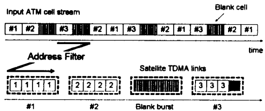
(그림 1) ATM/TDMA의 변환 과정 (Fig. 1) ATM/TDMA conversion system
