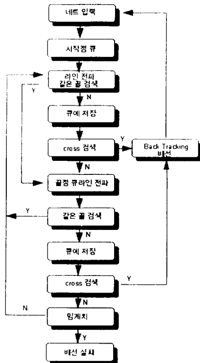
(그림 10) 개선된 그리드방식의 흐름도 (Fig. 10) Flowchart of improved grid method
