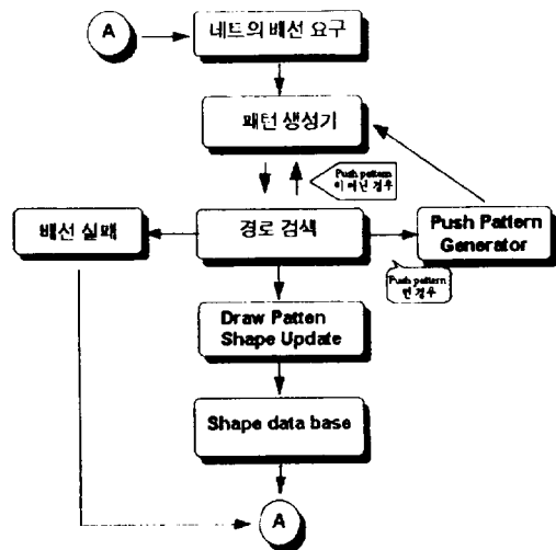
(그림 6) Shape based 패턴 라우터의 흐름도 (Fig. 6) Flowchart of the shape based pattern router
