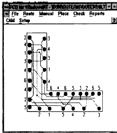
(그림 15) L-형 채널 실행 결과 (Fig. 15) Executed result on L-shaped channel
