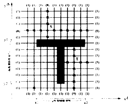
(b) 그리드를 적용한 초기 알고리즘 (b) Initial algorithm using grid
