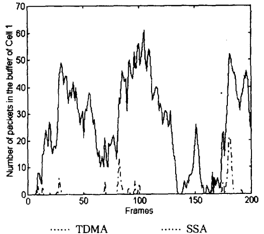
(그림 8) 높은 전송요구를 가진 셀의 버퍼 대기 패킷 (Fig. 8) Packets Wating in the Buffer on the High Transfer Demands
