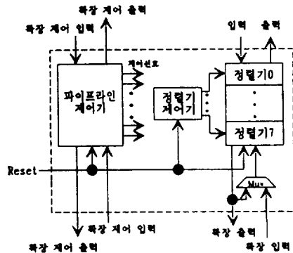
(그림 7) 확장형 리바운드 칩의 블록도 (Fig. 7) Block Diagram of a Expandable Rebound Chip
