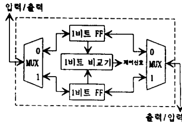
(그림 2) VLSI 정렬기의 기본셀 (Fig. 2) Basic Cell of VLSI Sorter
