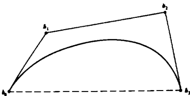
(그림 1) 베지어 곡선과 제어다각형
