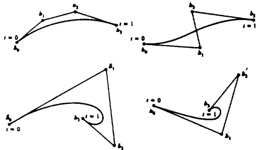
(그림 2)여러가지 3차 베지어 곡선
