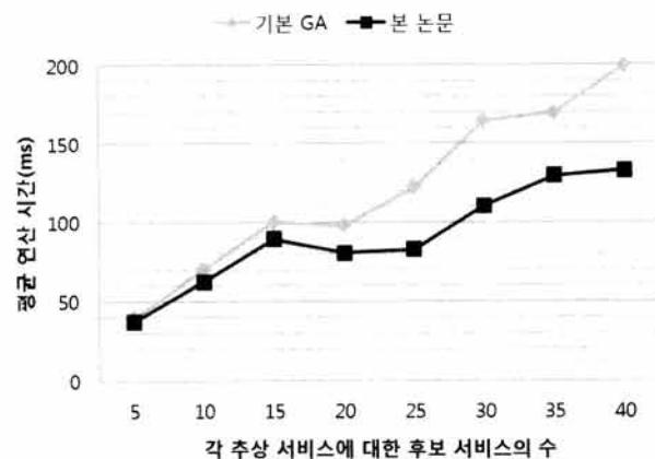
그림 5. 후보 서비스에 따른 연산시간 Fig. 5. Computational time as candidate services increases
