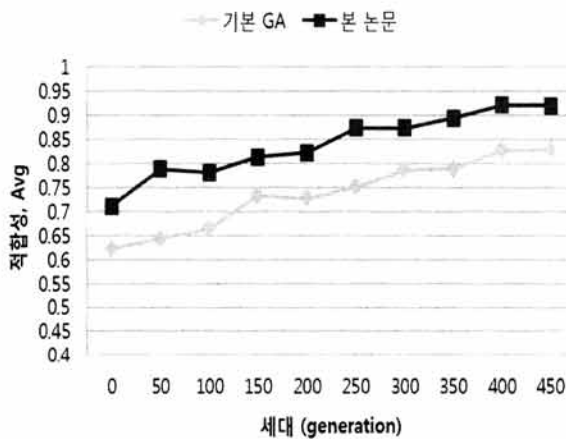
그림 6. 세대에 따른 평균 적합성 Fig. 6. Average fitness as generation increases
