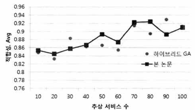
그림 8. 추상 서비스 변화에 따른 적합성 Fig. 8. Average fitness as abstract services increases
