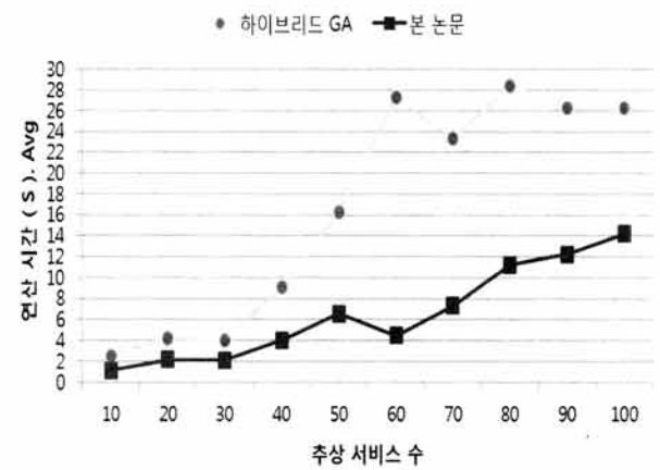
그림 7. 추상 서비스에 따른 연산시간 Fig. 7. Computational time as abstract services increases
