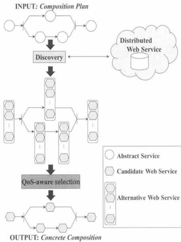
그림 1. QoS 고려 합성 서비스 선택과정 Fig. 1. A QoS-aware selection process for composition service
