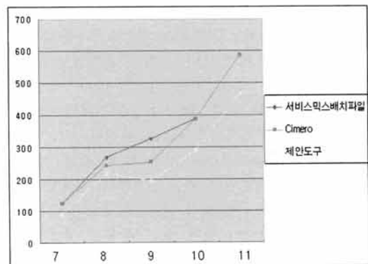
(그림 18) 실험조건 2의 패키징 효율성 실험
