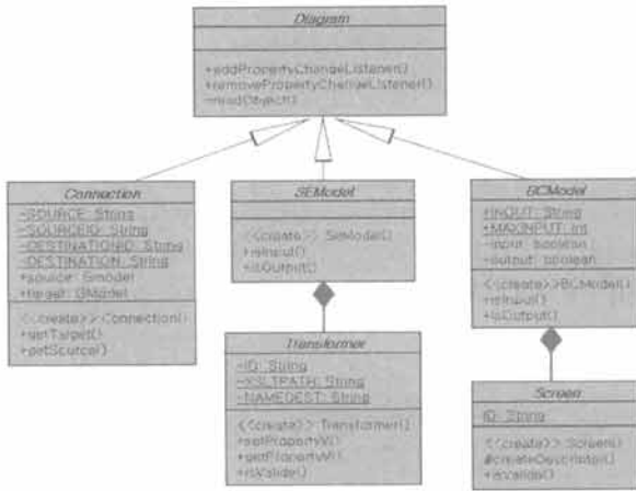
(그림 6) 모델링 클래스 다이어그램
