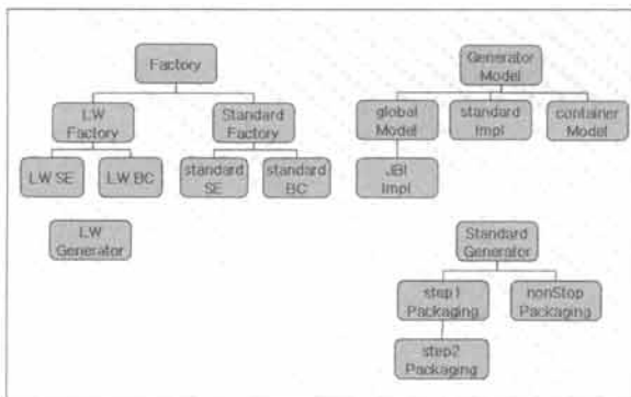
(그림 7) 패키징기능의 클래스패키징구조
