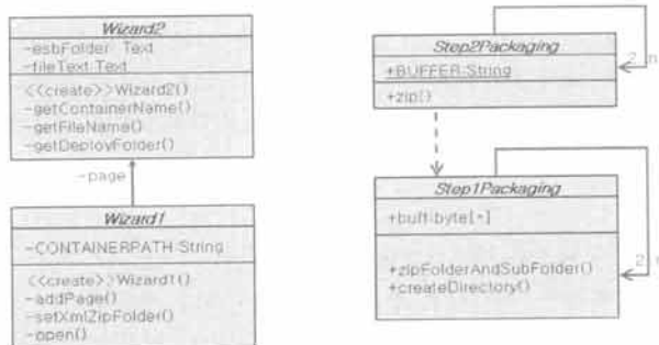
(그림 10) 서비스배포와 컴포넌트관리 클래스 다이어그램
