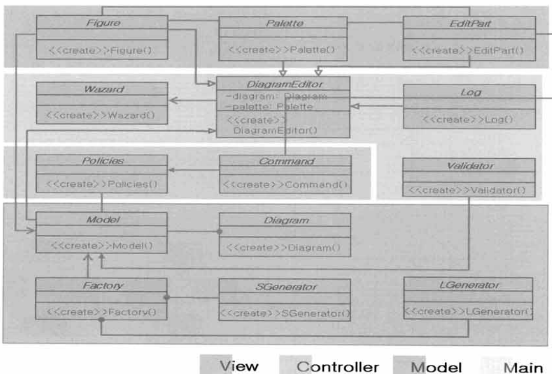
(그림 4) 컴포넌트배치도구의 구조
