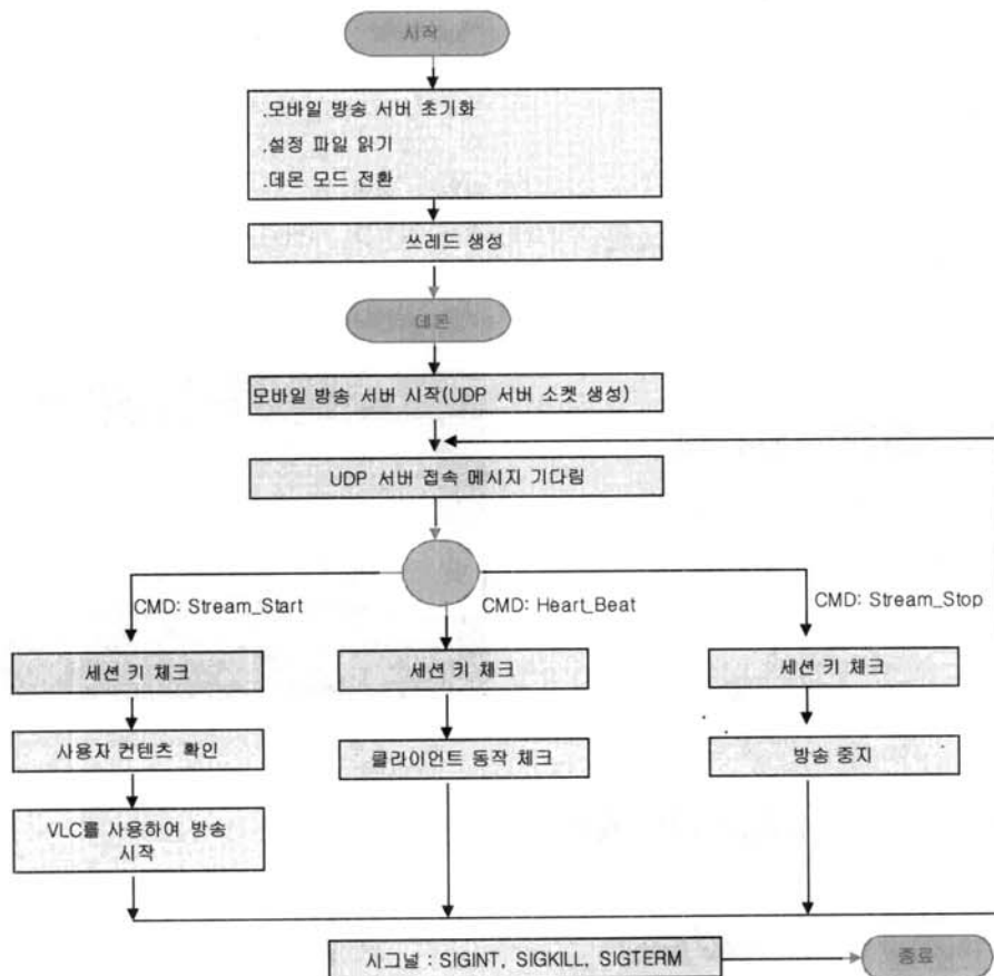
(그림 5) 모바일 방송 서버의 동작 흐름도
