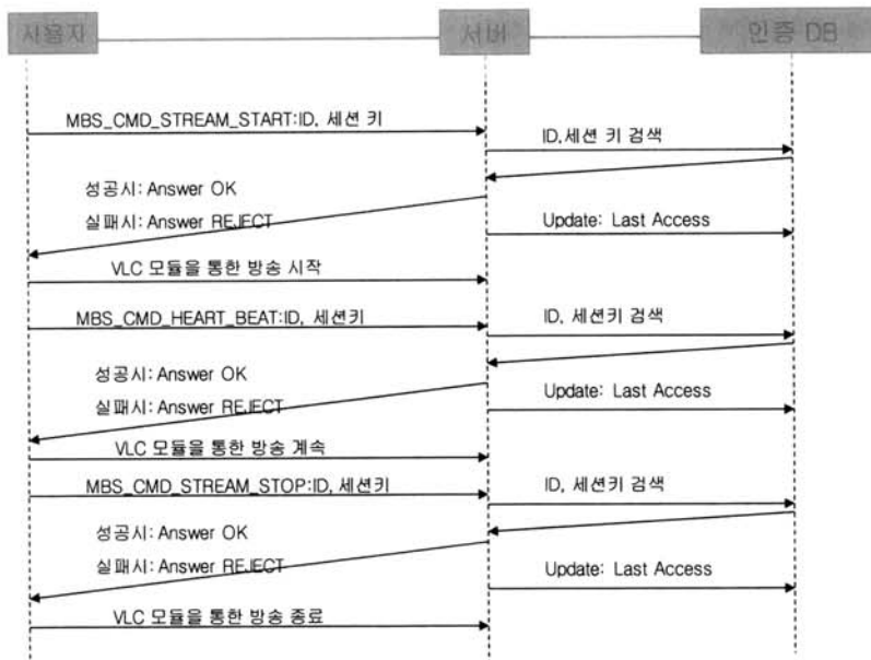
(그림 6) 모바일 방송 클라이언트와 서버간의 통신 절차
