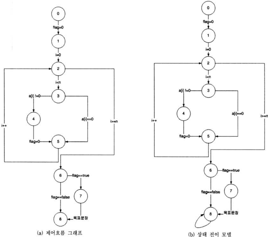
(그림 5) 함수 'flagProc4'의 제어 흐름 그래프와 상태 모델
