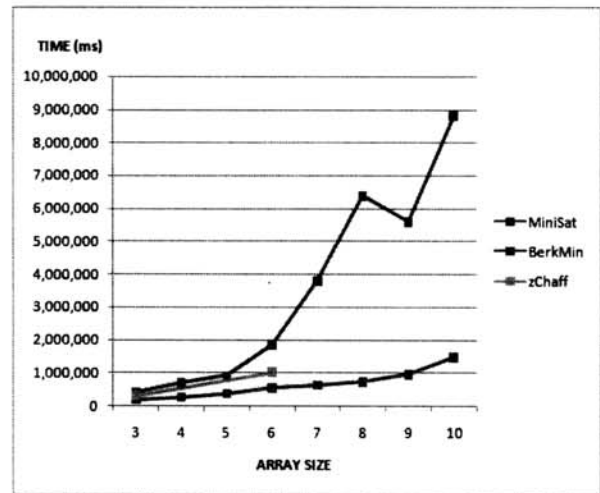
(그림 15) SAT 해결기에 따른 성능 비교
