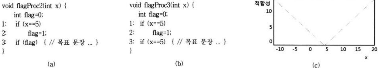
(그림 2) (a) 예제 프로그램 (b) 변환된 예제 프로그램 (c)적합성 함수
