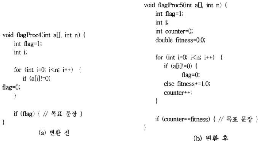
(그림 3) 반복문 내에서 플래그 변수 정의 예제 프로그램
