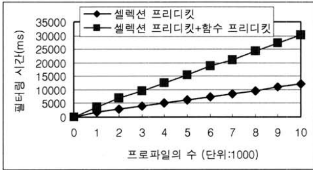
(그림 10) 선택선 및 함수 프리디킷에 대한 필터링 비교
