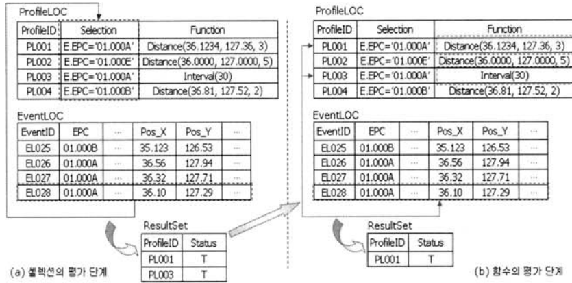
(그림 8) 이벤트 필터링의 과정
