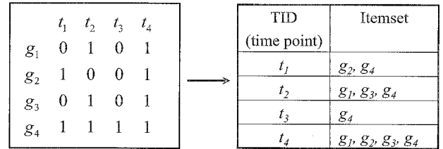
(그림 4) 유전자 배열로부터의 트랜잭션 생성 과정
