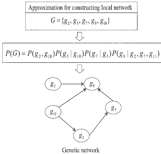
(그림 14) 유전자 조절 네트워크 구성 예
