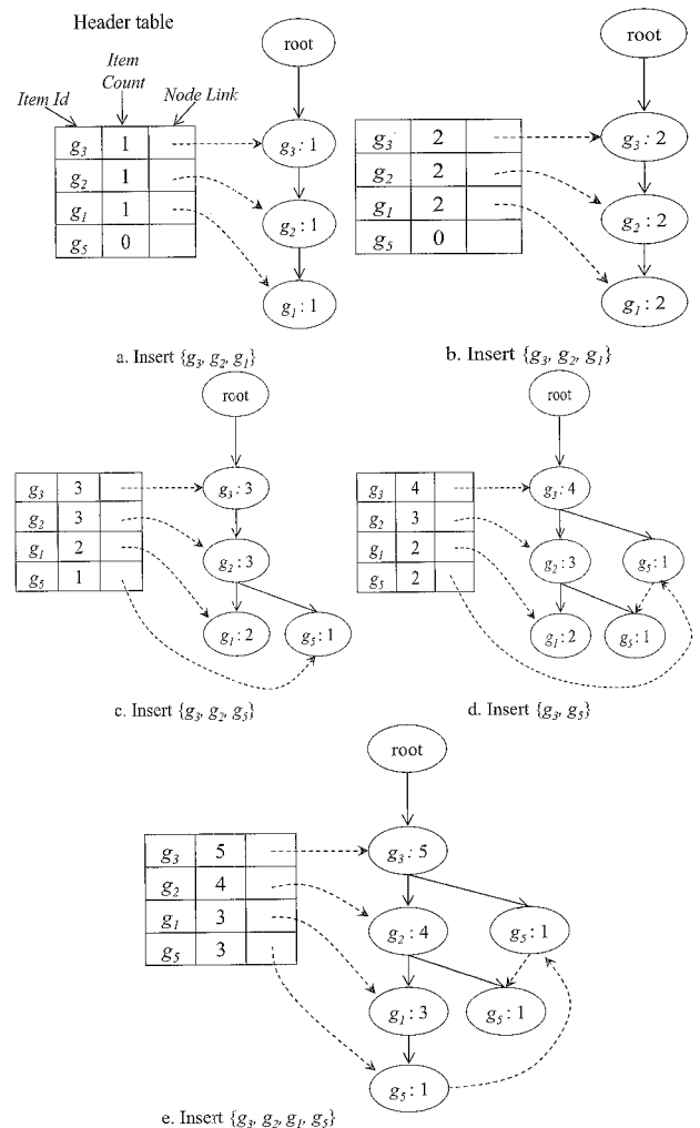
(그림 7) FP-tree의 구성과정
