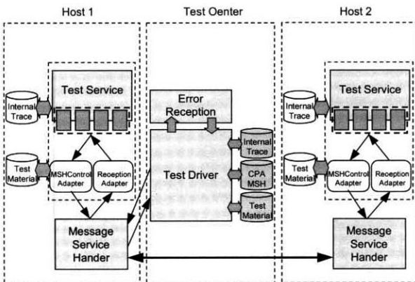
(그림 7) 상호운용성 검증을 위한 시스템 구성도
