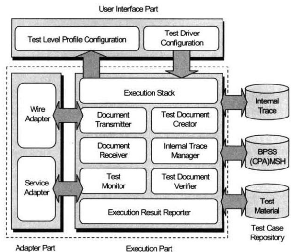
(그림 1) 테스트 드라이버 구성도
