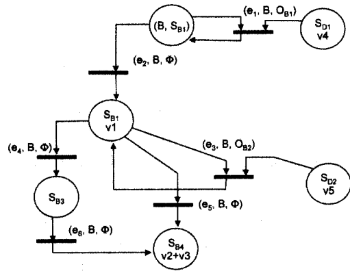
(그림 13) 객체 B의 CPN
