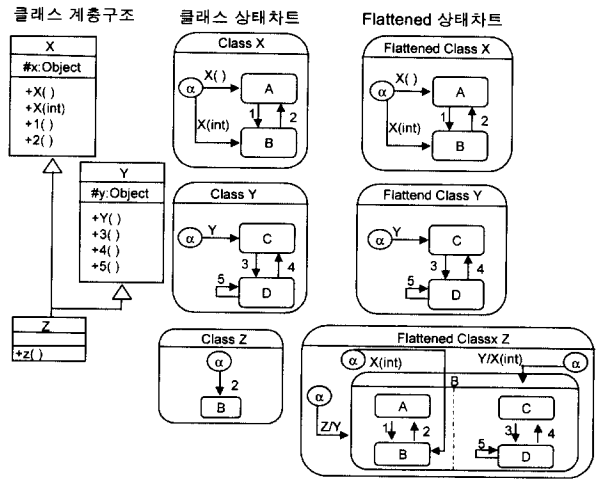
(그림 4) 평탄화된 상태차트 뷰(상속만 존재하는 경우)
