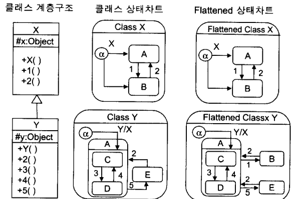
(그림 5) 평탄화된 상태차트 뷰(재정의 있는 경우)
