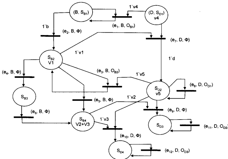
(그림 15) 객체 B와 D 상호작용의 단일 CPN
