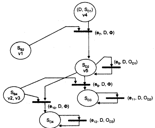
(그림 14) 객체 D의 CPN
