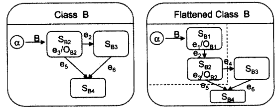
(그림 8) 클래스 B의 상태차트 다이어그램과 평탄화된 상태차트 다이어그램
