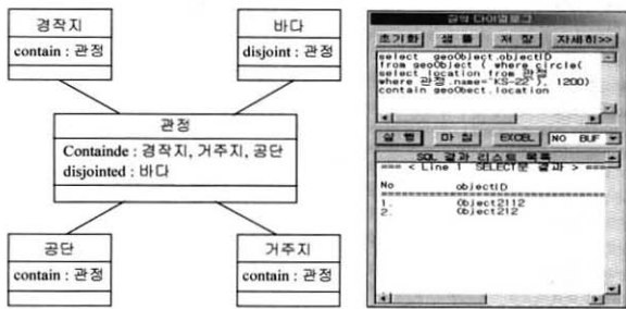
(a) 지리-객체 클래스계층구조 (b) 위상 관계 연산을 위한 ZEUS/SQLX
