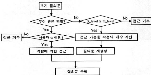
(그림 3) MAC과 RBAC 모듈 처리 순서도
