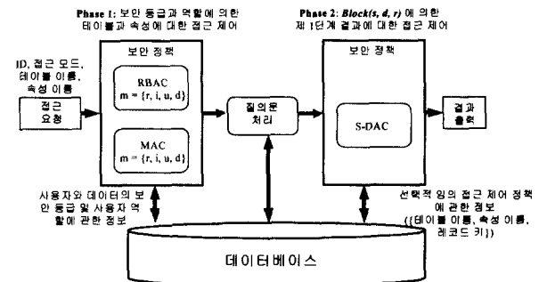
(그림 2) 시스템 구조
