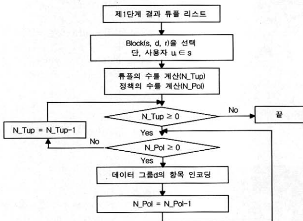
(그림 4) S-DAC 모듈 처리 순서도
