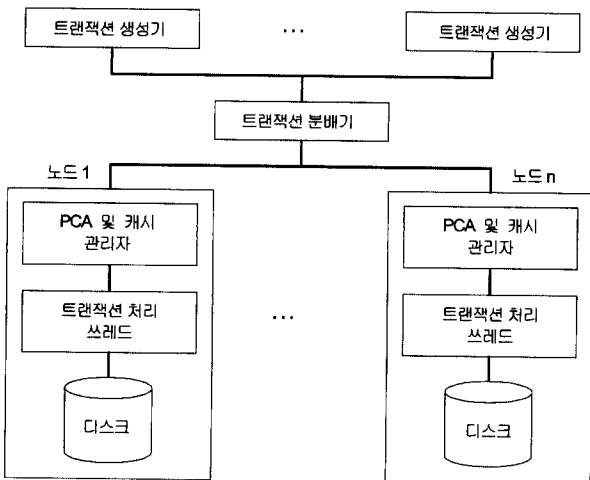
(그림 10) 분산 트랜잭션 처리 시스템의 시뮬레이션 모델
