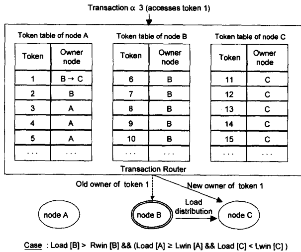
(그림 8) 다른 노드의 토큰을 보유한 경우(부하가 LWin 이하인 노드로 분산)
