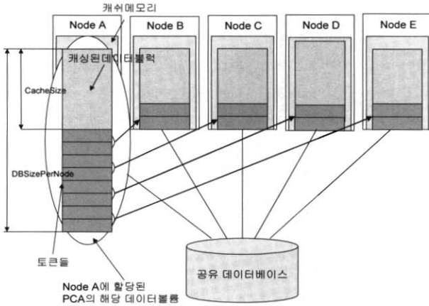
(그림 4) 트랜잭션이 PCA 노드 A에게 집중될때의 토큰의 분배
