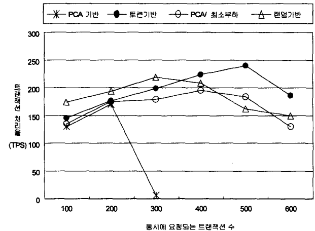
(그림 12) 편중된 데이터 참조의 경우 트랜잭션 처리율
