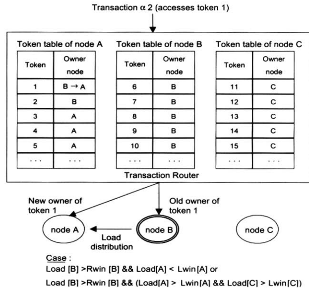
(그림 7) 다른 노드의 토큰을 보유한 경우(PCA 노드로의 분산)
