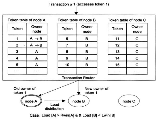
(그림 6) 노드가 자신의 토큰만을 보유한 경우
