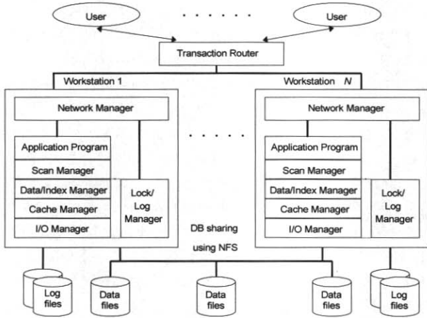
(그림 1) 분산 트랜잭션 시스템의 전체구조
