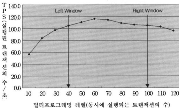
(그림 3) 단일 트랜잭션 시스템의 TPC-B 벤치마크 성능 분석 결과
