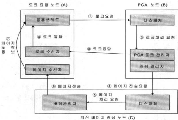
(그림 2) PCA 기반의 분산 로킹 처리 과정
