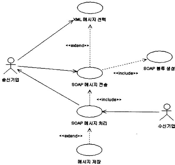
(그림 4) 유즈케이스 다이어그램
