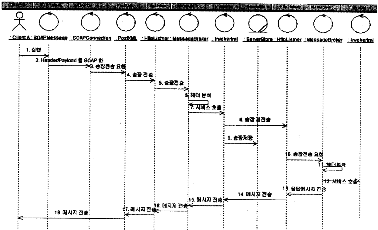
(그림 5) 순차 다이어그램
