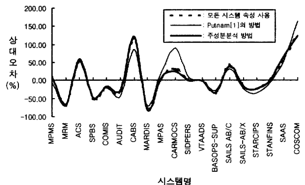
(그림 6) 개발 난이도 추정 상대오차
