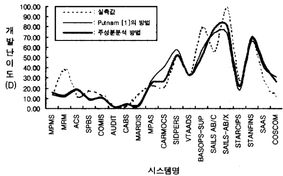
(그림 4) 개발 난이도 추정
