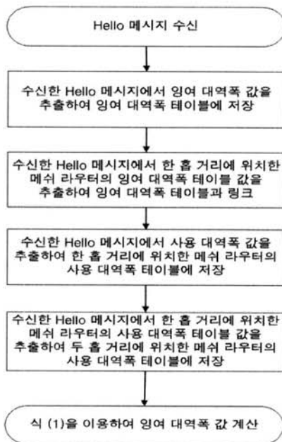
(그림 4) 이웃 노드들의 영어 대역폭 정보 저장 및 영어 대역폭 계산 알고리즘
