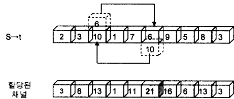
(그림 12) CAP3알고리즘의 이웃해 생성방법
