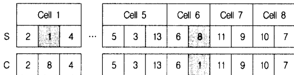
(그림 11) n세대의 해(s)와 선택된 이웃해(c')
