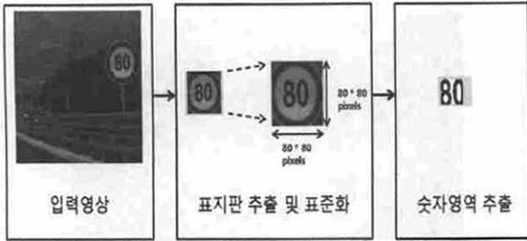
(그림 3) 속도 표지판 검출 예
