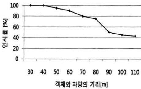
(그림 13) 거리별 인식률 결과
