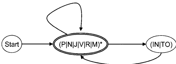
(그림 2) 유사 표현구 인식을 위한 상태 전이도
