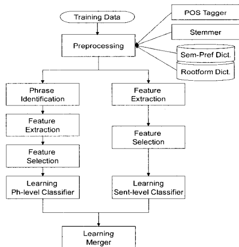
(그림 4) 문장 분류기 전체 흐름도
