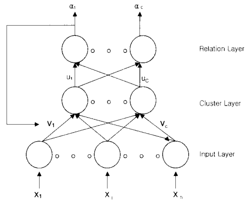
(그림 2) 비교사 퍼지 학습신경망
