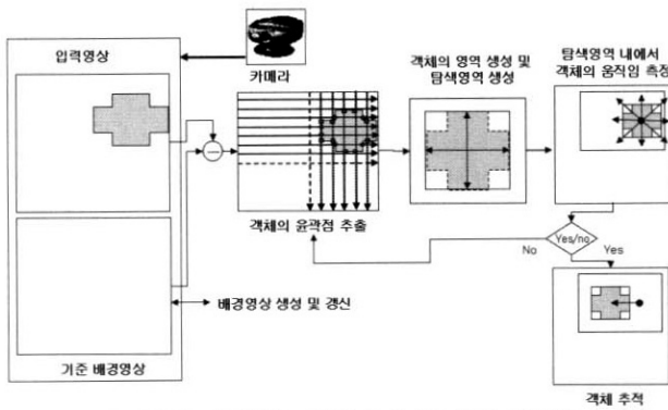
(그림 4) 제안하는 객체 추출 및 추적 시스템
