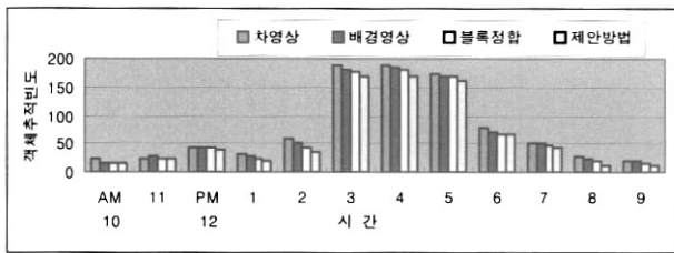
(그림 13) 객체 추적 빈도수 측정결과
