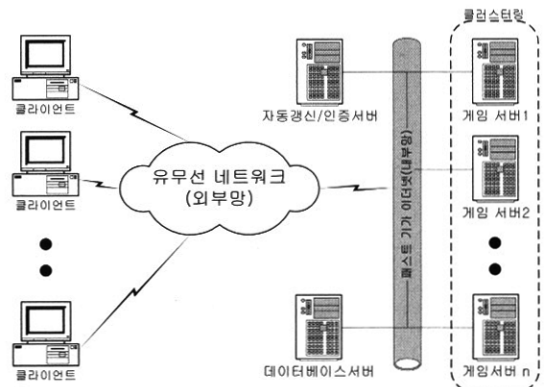
(그림 3) 비 대칭형 다중 게임서버 구조
