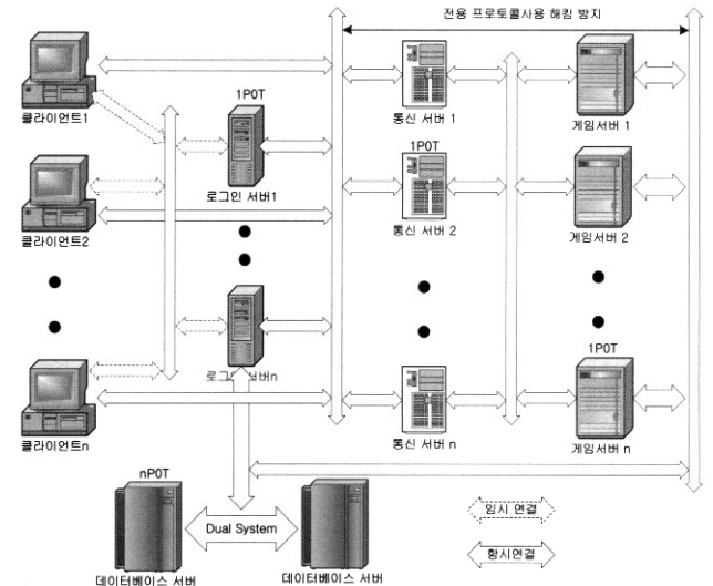
(그림 7) 제안된 비대칭 분산형 다중 서버구조
