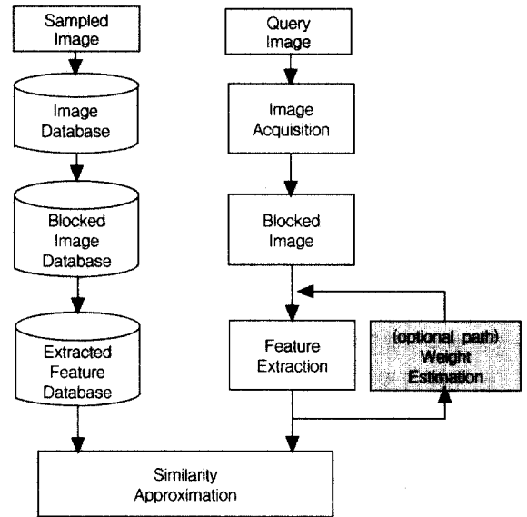
(그림 1) 제한한 알고리즘에 대한 흐름도
