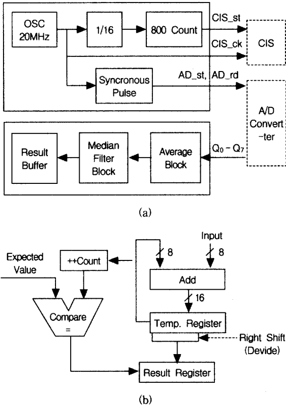
(그림 7) PLD의 구성 : (a) 전체 블록도, (b) 평균화 블록도
