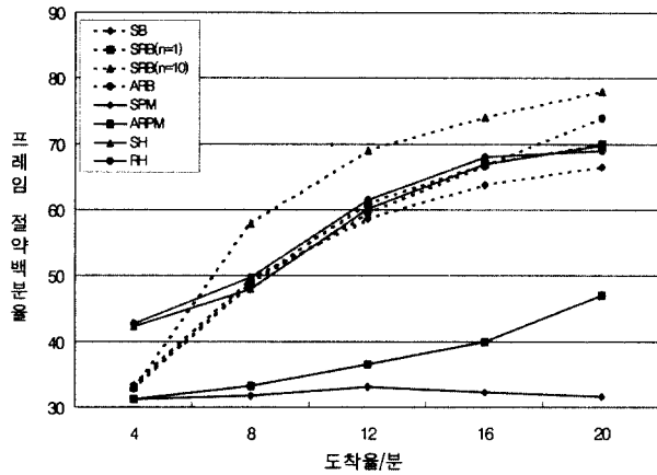
(그림 8) 비디오 요청 도착율에 따른 각 정책별 프레임 절락 백분율
