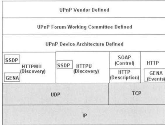
(그림 1) UPnP 프로토콜 스택
