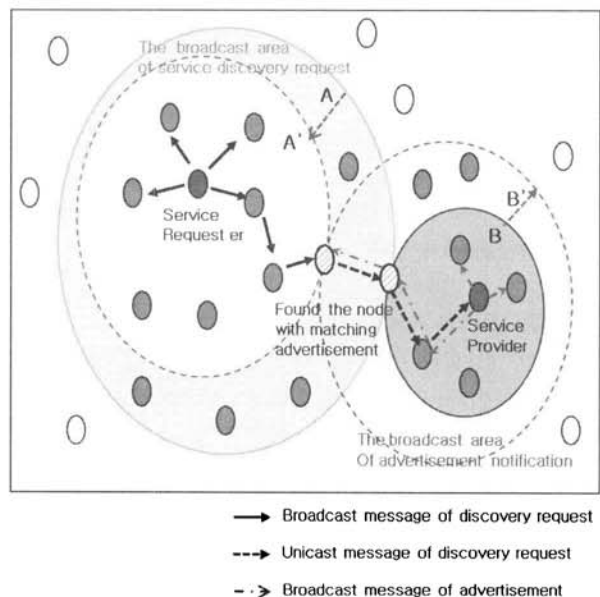
(그림 3) fSSDP의 서비스 발견 및 광고 영역의 상태 변화 예
