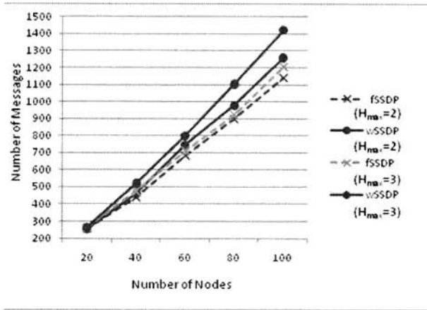
(그림 10) 실험을 통한 wSSDP와 flexible SSDP의 서비스 발견 및 광고 메시지 발생에 따른 메시지 오버헤드 비교
