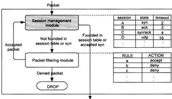
(그림 7) 세션 관리 시스템의 동작도
