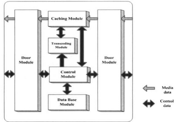
(그림 2) Media Proxy Block diagram
