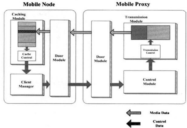
(그림 4) 전송 메커니즘
