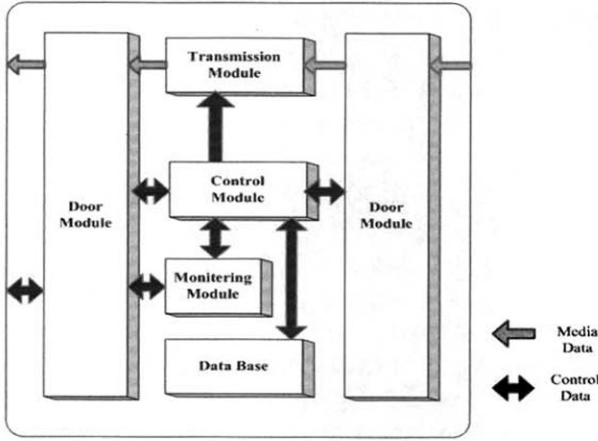
(그림 3) Mobile Proxy Block diagram
