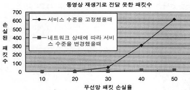
(그림 12) 무선망 손실률에 따른 재생기로의 패킷 손실
