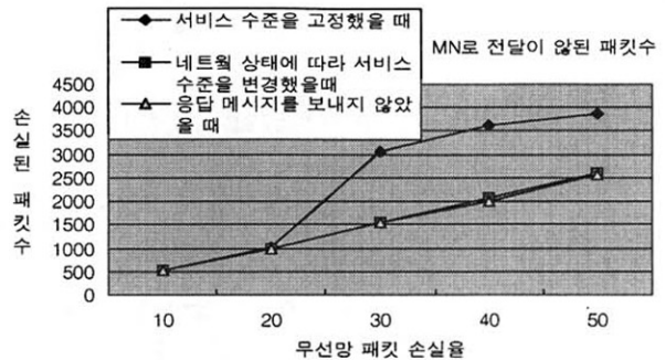
(그림 11) 무선망 손실률에 따른 MN로 전달이 안된 패킷수
