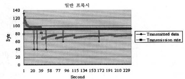
(그림 8) 일반 프록시를 사용하였을 때 MN로 전송된 미디어 데이터
