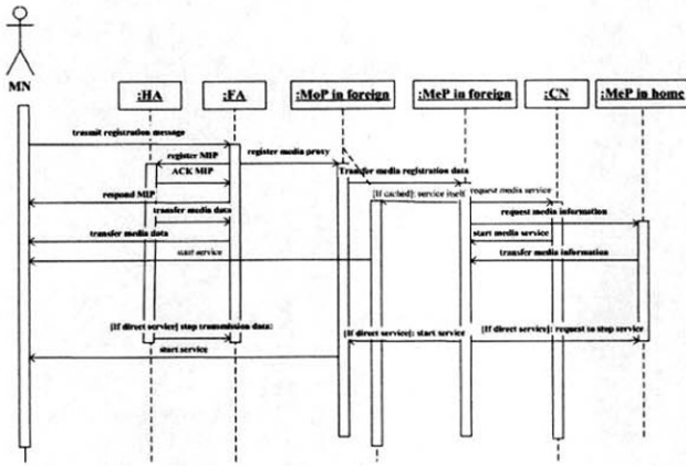
(그림 5) Proxy handoff sequential diagram
