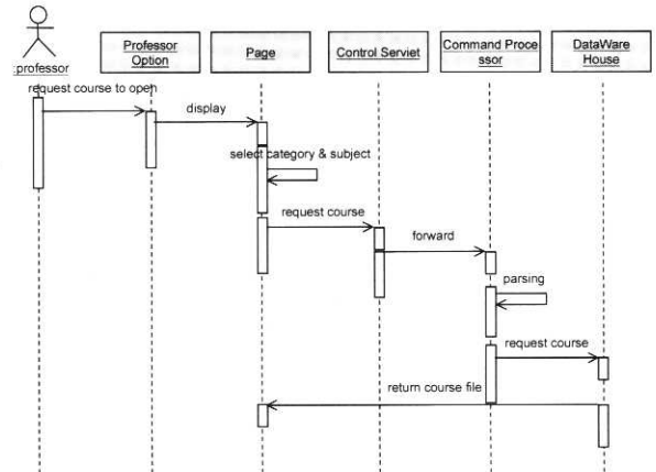
(그림 16) 객체 저장소에서 코스 얻기 시퀀스 다이어그램
