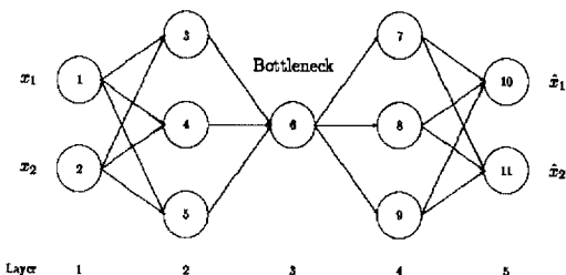
(그림 3) NLPCA를 위한 5-layer feed-forward 신경망 구조
