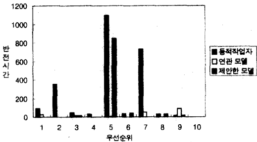
(그림 11) 우선 순위 반전시간(단위:ms)
