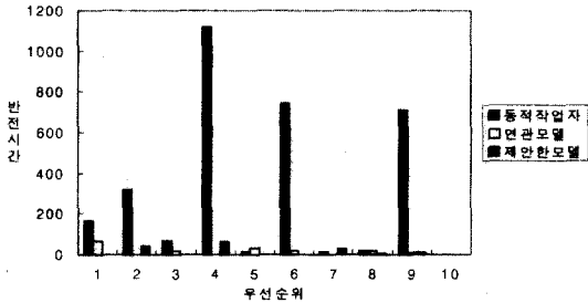
(그림 13) 우선 순위 반전시간 (단위:ms)
