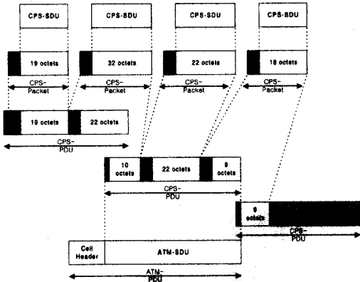
(그림 3) CPS-SDU를 ATM셀로의 다중화 및 패키징과정
