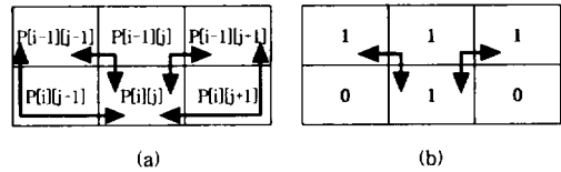
(그림 6) 세선화척도 (a)세선화척도를 위한 이웃관계 (b)thinness( P[i][j] )=2
