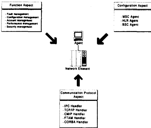
(그림 2) TMN 에이전트의 관찰측면
