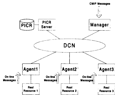
(그림 4) Simulation 환경
