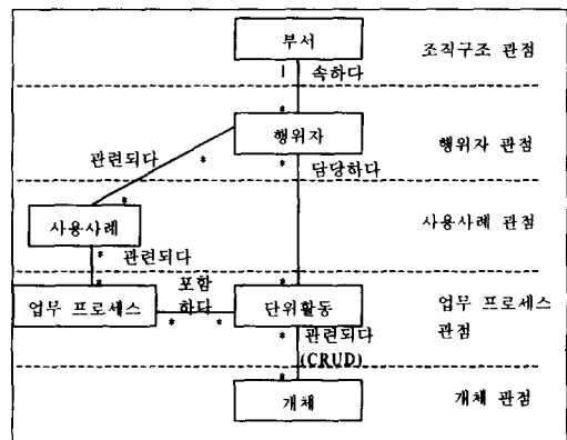
(그림 2) 업무 시스템의 메타 모형
