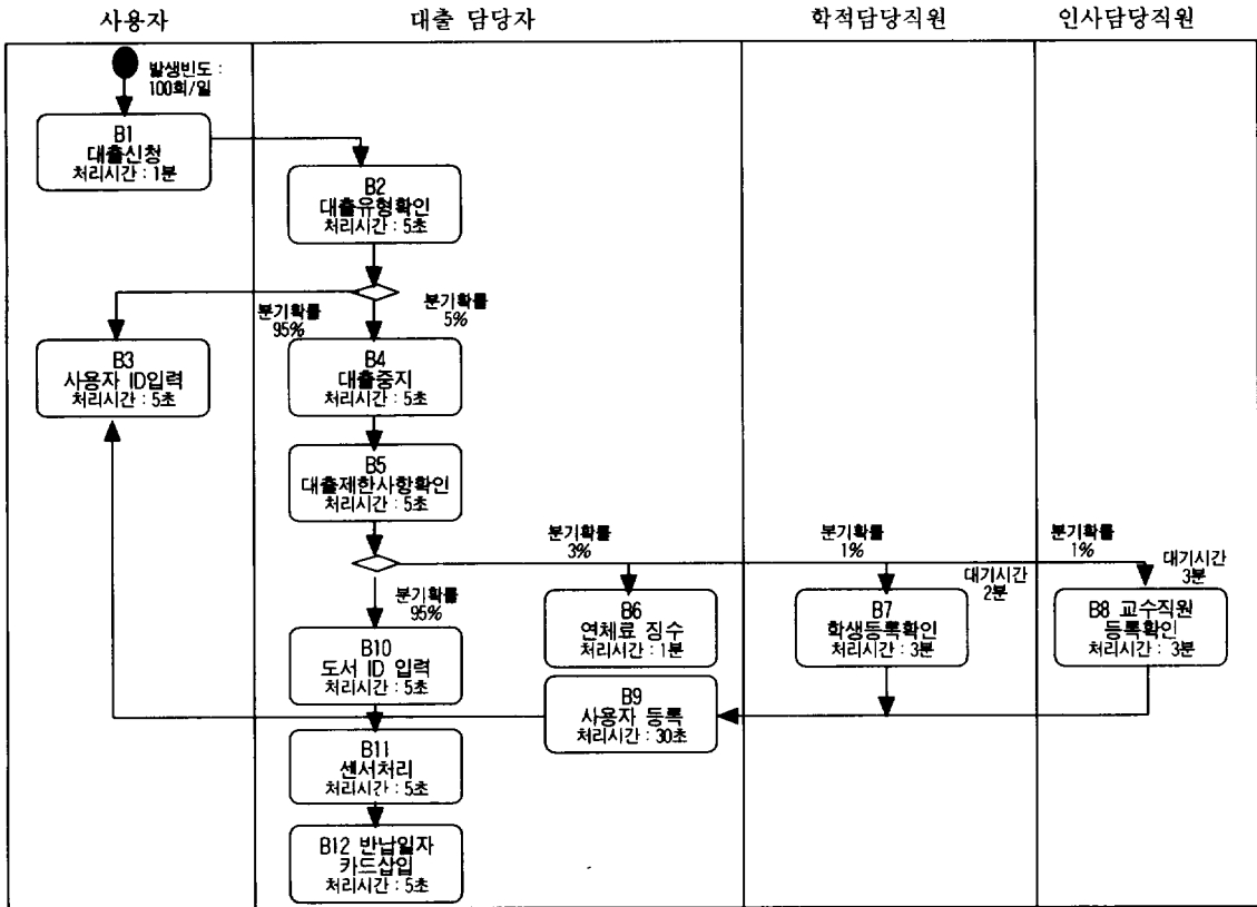
(그림 7) 대출 사용사례의 활동도
