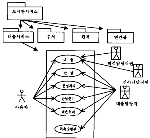
(그림 6) 사용사례 관점을 표현하는 사용사례도
