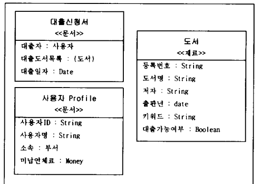
(그림 5) 개체 관점을 표현하는 클래스도
