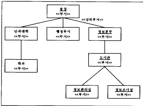
(그림 4) 조직 관점을 표현하는 클래스도
