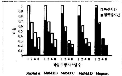
(그림 11) 통신시간이 전체 성능에 미치는 영향
