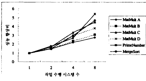
(그림 7) Speedup 비교
