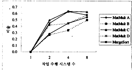
(그림 10) 통신시간 중첩률
