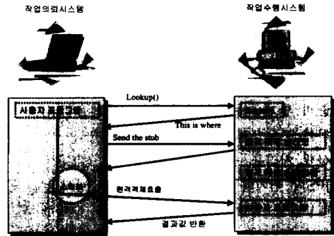
(그림 6) 원격 메소드 호출 메카니즘
