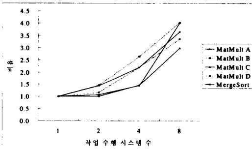
(그림 9) 통신 오버헤드 비율
