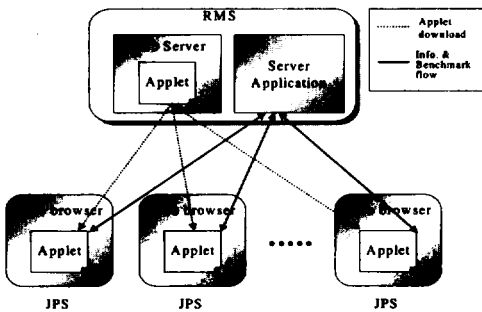
(그림 4) 자원 중계 관리 시스템의 구성
