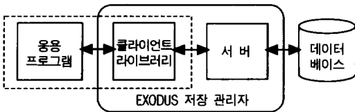
(그림 3) EXODUS 저장 관리자
