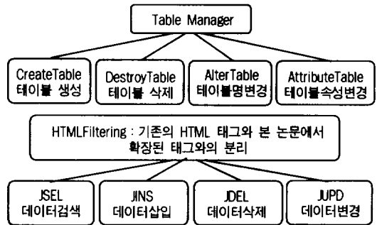
(그림 4) UCM 프로시저
