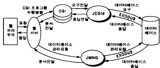
(그림 1) UCM 시스템
