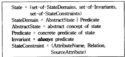
(그림 4) 상태 도메인 표현 (Fig. 4) Representation of State Domain
