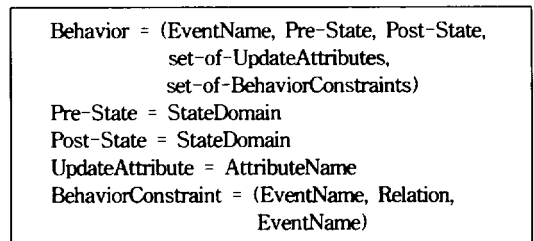
(그림 5) 행위 표현 (Fig. 5) Representation of Behavior
