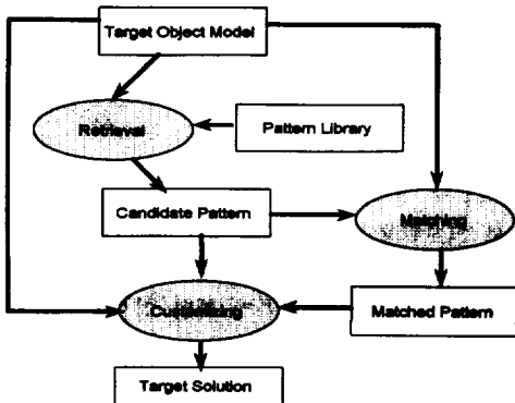
(그림 9) 재사용 시스템의 전체 흐름도 (Fig. 9) Flow Diagram of Reuse System
