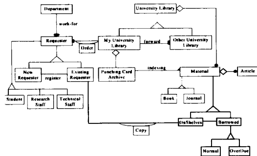
(그림 13) 개선된 객체 모델 (Fig. 13) Revised Object model
