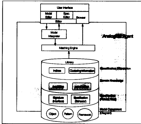
(그림 10) Analogical Agent의 구조 (Fig. 10) Architecture of Analogical Agent
