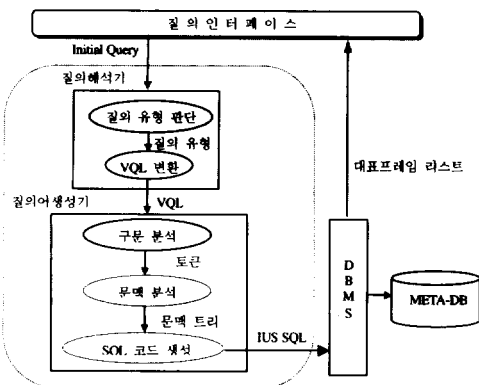
(그림 2) 비디오 검색기의 구조 (Fig. 2) Architecture of Video Retrieval Engine
