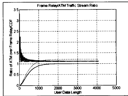
(그림 4) 실제 대역 비와 CDF (Fig. 4) Actual bandwidth ratio and CDF
