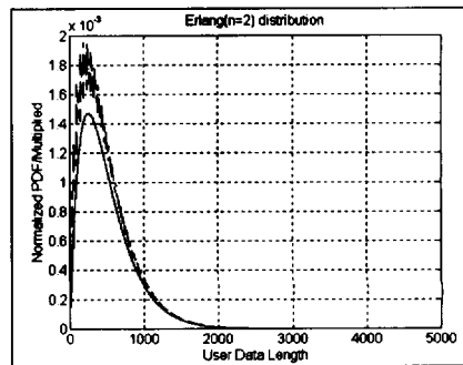
(그림 5) PDF 및 BWR 곱의 PDF 예(평균=500) (Fig. 5) An example for PDF and multiplied PDF (average=500)
