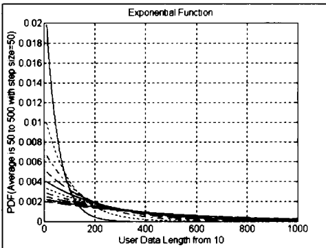
(b) 지수 함수 분포 (b) Exponential distribution
