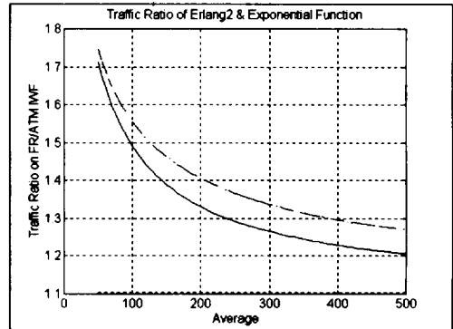
(그림 7) 평균에 따른 대역 비 (Fig. 7) Bandwidth ratio in accordance with average
