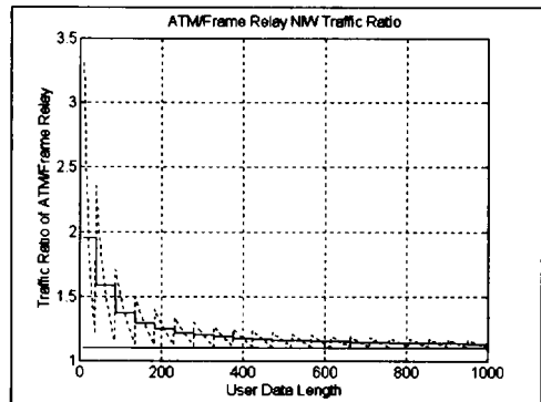
(그림 1) 프레임 길이에 따른 대역 비율 BWR (Fig. 1) Bandwidth ratio BWR in accordance with frame length
