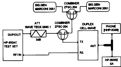
(그림 4) 시험 구성도 (Fig. 4) Test configuration
