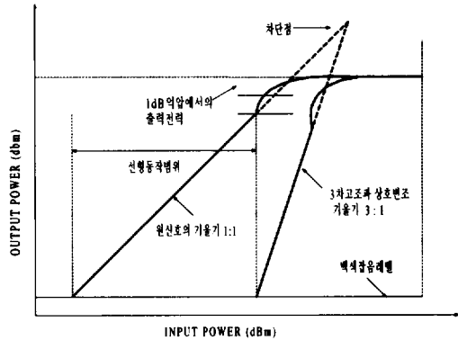
(그림 3) 선형영역과 3차고조파 차단점
