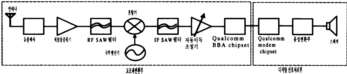
(그림 1) 수신기의 구성도 (Fig. 1) Configuration of receiver
